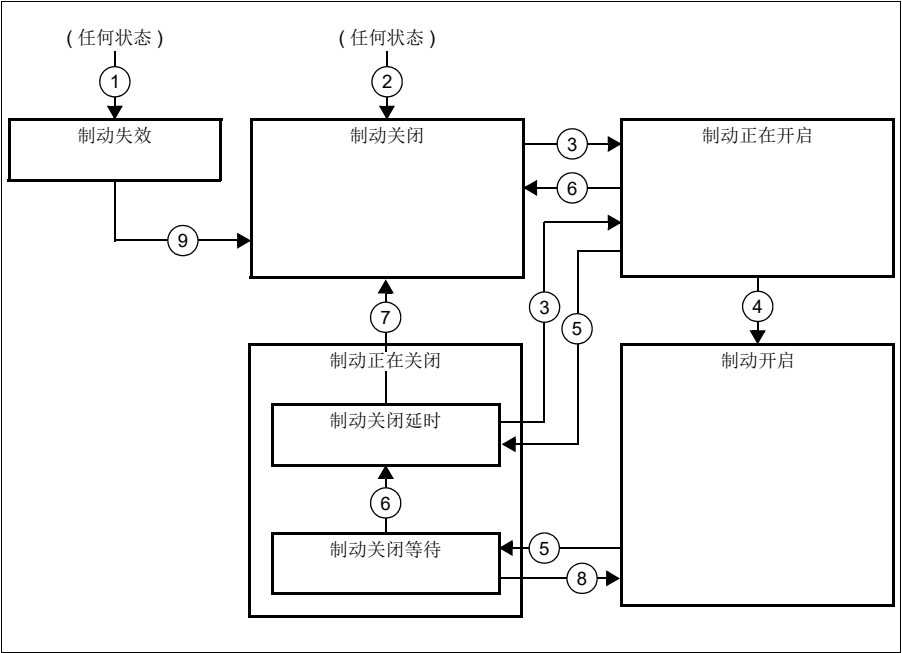
制动状态图表
