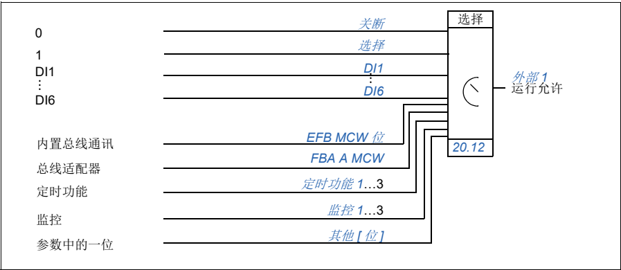
图示：外部 1 的运行允许源
